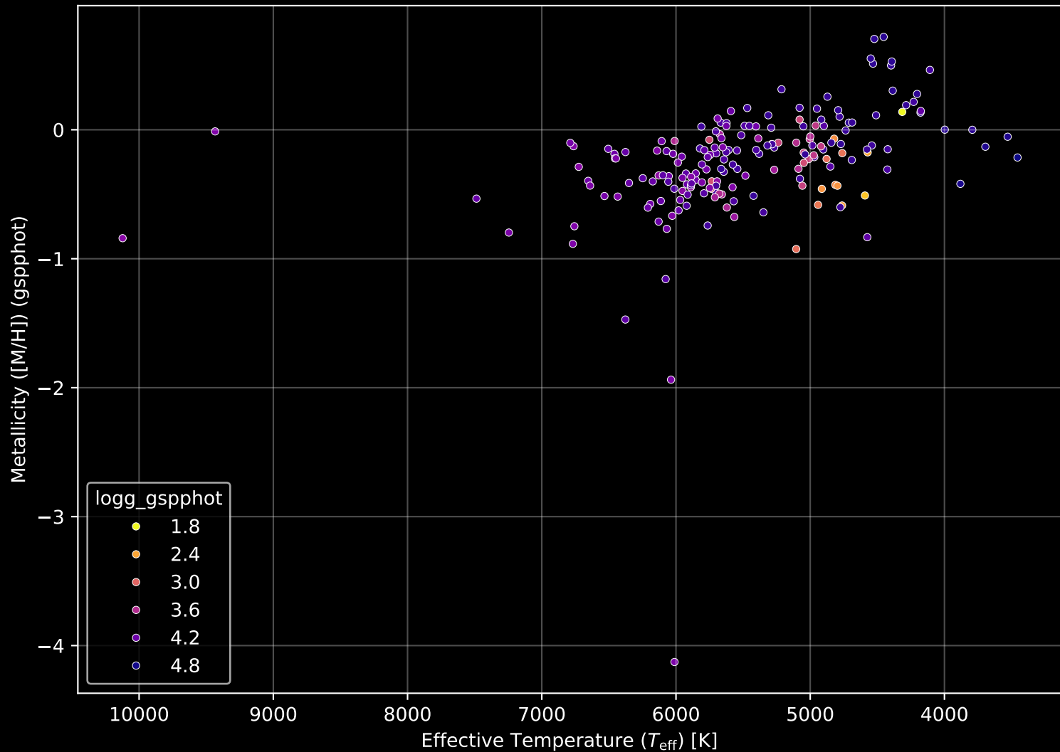
APOGEE DR17 Field: [185+57_MGA] Stellar Population Parameters (n= 192)
